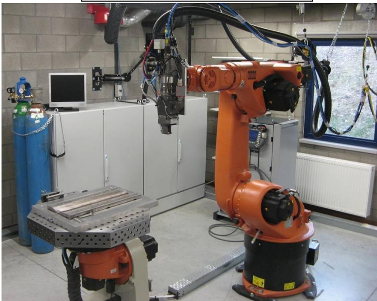
Robot KUKA 6 Axes + table 2 axes
